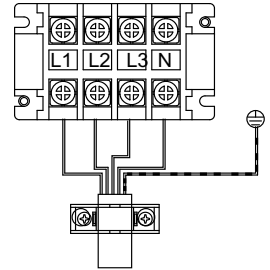
12-15 3Ph
