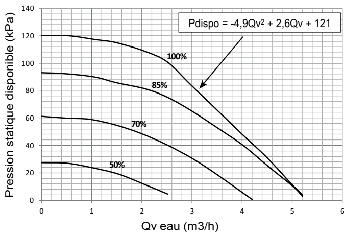
GeoCIATTM Power 50H(T) - 65HT
