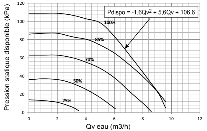
GeoCIATTM Power 90HT - 120HT
