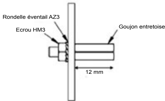
Détails entretoises métallique (vue de côté)
