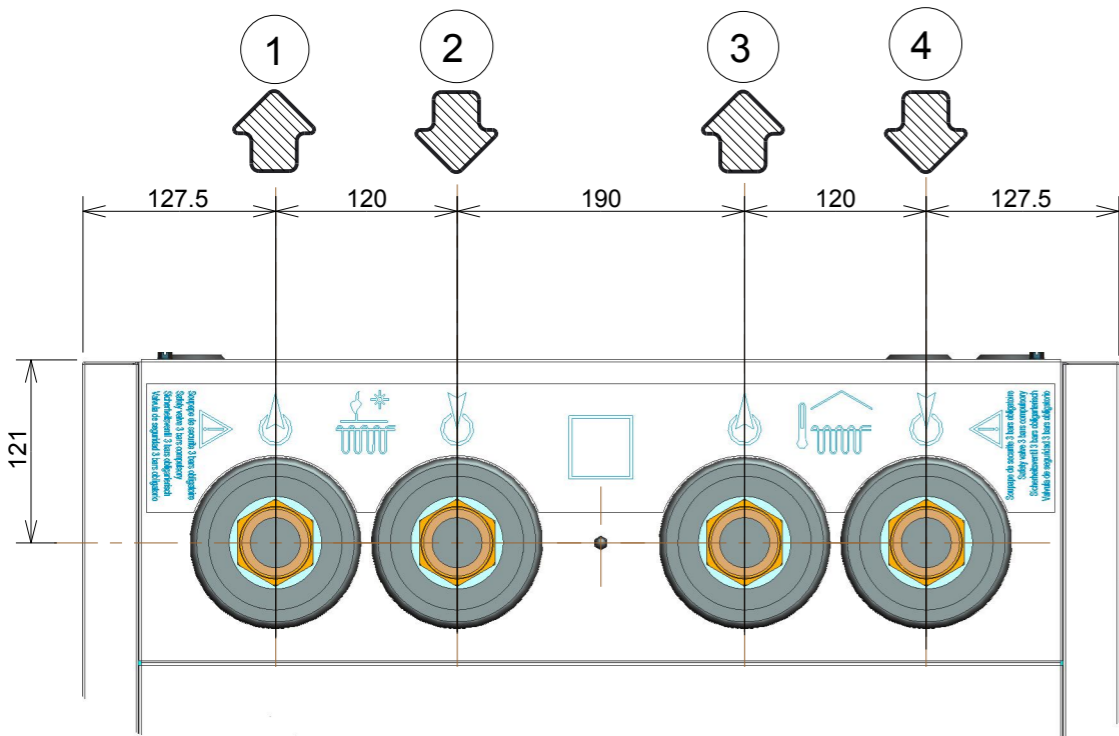
A Détail A Ech. 0.200
