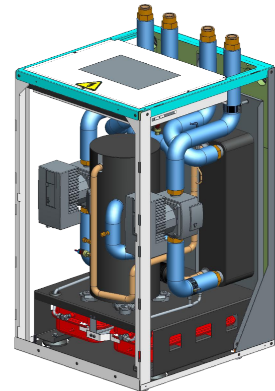
Vue ISO (Non carrossée) (Without casing) Ech. 0.075
